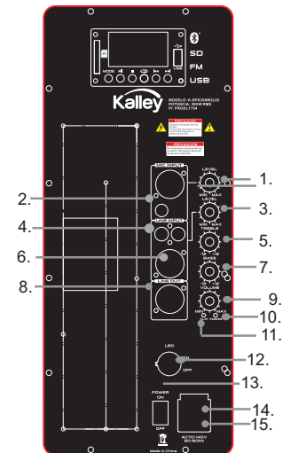
VISTA TRASERA
